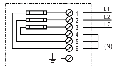
Fig.6 Typ: EZ-3600 400 V 3~
