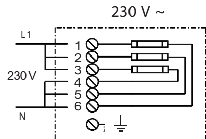
Fig.5 Typ: EZ-3600
